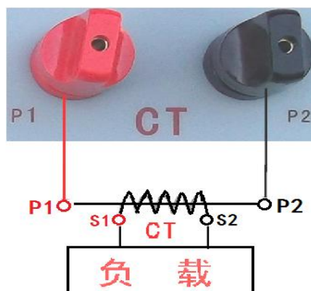
图 15、CT 一次通流接线图
