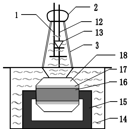
图 2：单台耐压试验装置内部结构图
