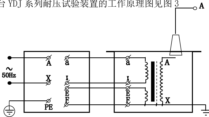
图 3: 单台 YDJ 系列油浸式工频耐压试验装置原理图
